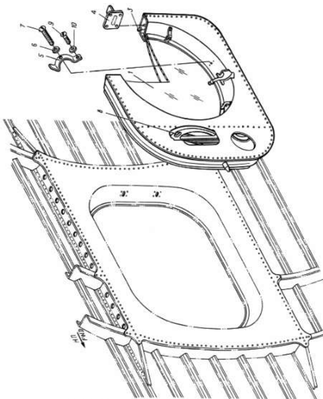
Рис. 3. КРЫШКА БОКОВОГО АВАРИЙНОГО ВЫХОДА ПРАВА, (ЛЕВ.) Fig. 3. SIDE EMERGENCY EXIT COVER RH (LH)
